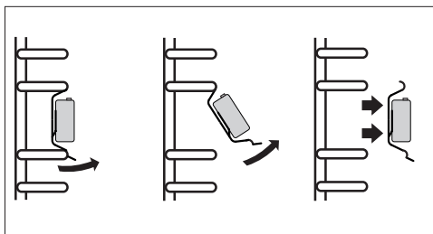
Wymowanie prowadnic teleskopowych
