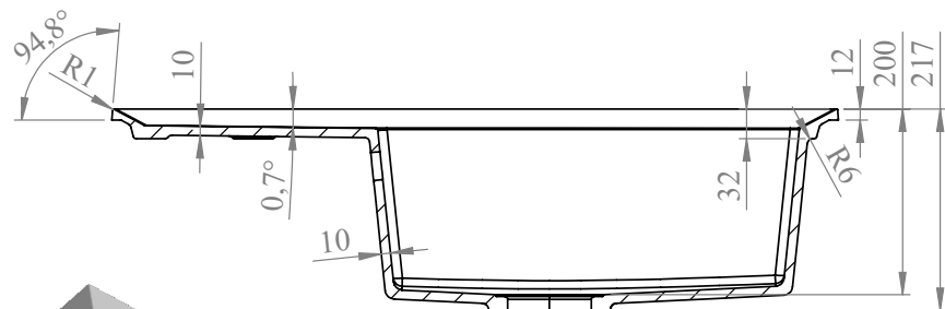
PRZEKRÓJ N-N SKALA 1 : 8
