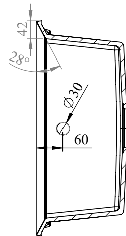
PRZEKRÓJ M-M SKALA 1 : 8
