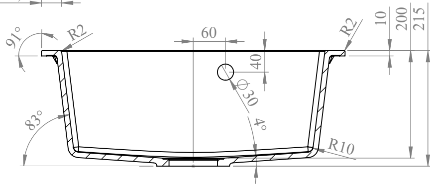
PRZEKRÓJ H-H SKALA 1 : 7
