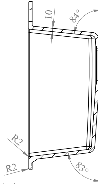
PRZEKRÓJ G-G SKALA 1 : 7
